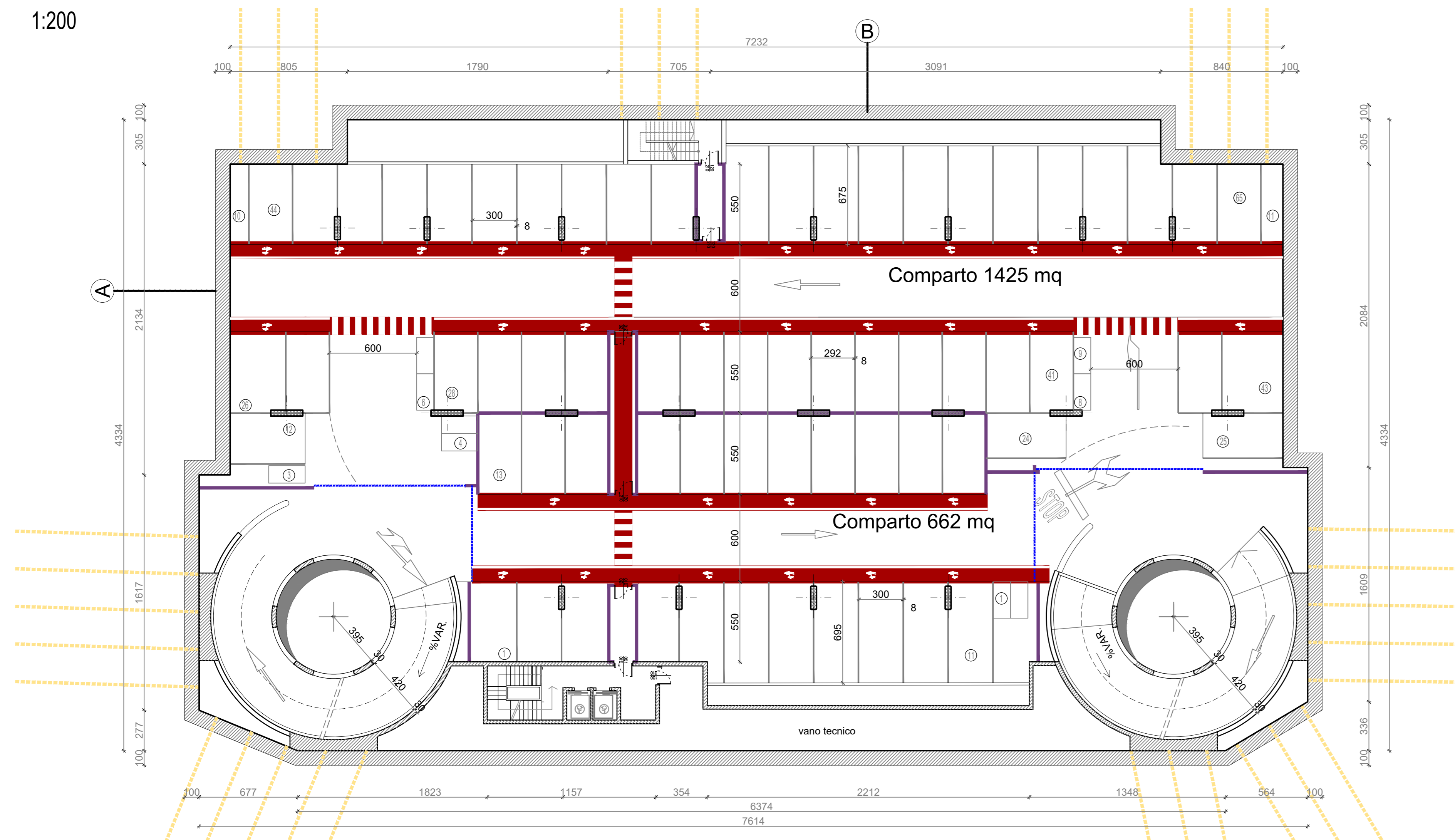
GRUNDRISS: 6. UNTERGESCHOSS PIANTA: PIANO -6 1:200
