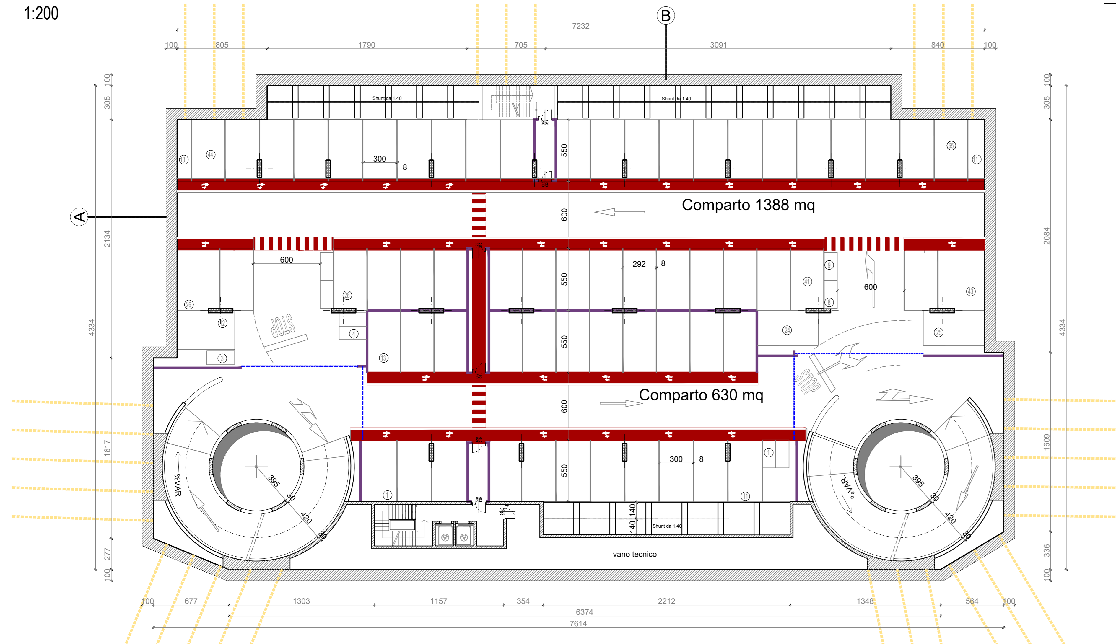
GRUNDRISS: 4. UND 5. UNTERGESCHOSS PIANTA: PIANO -4 E PIANO -5 1:200
