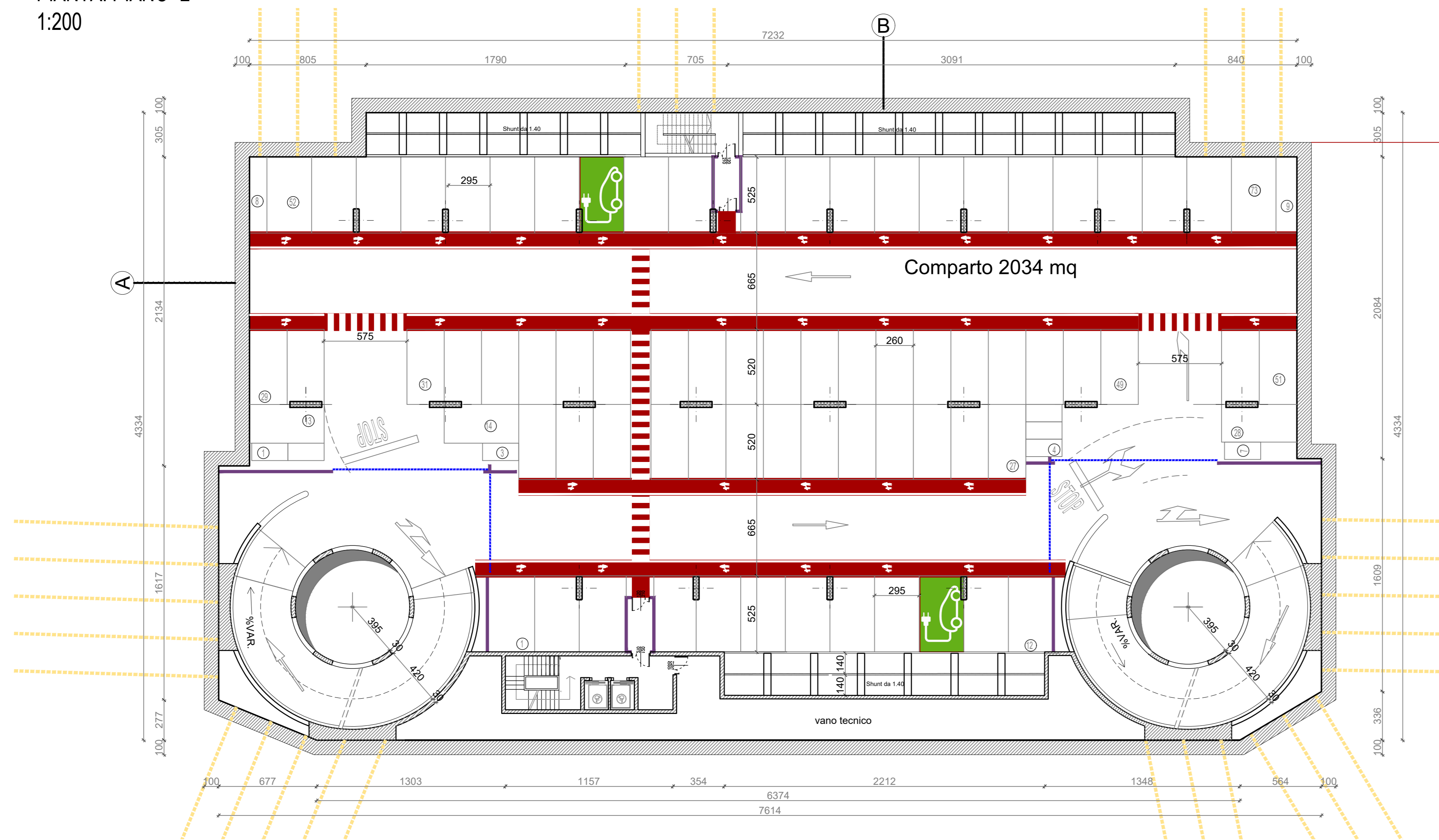
GRUNDRISS: 3. UNTERGESCHOSS PIANTA: PIANO -3 1:200
