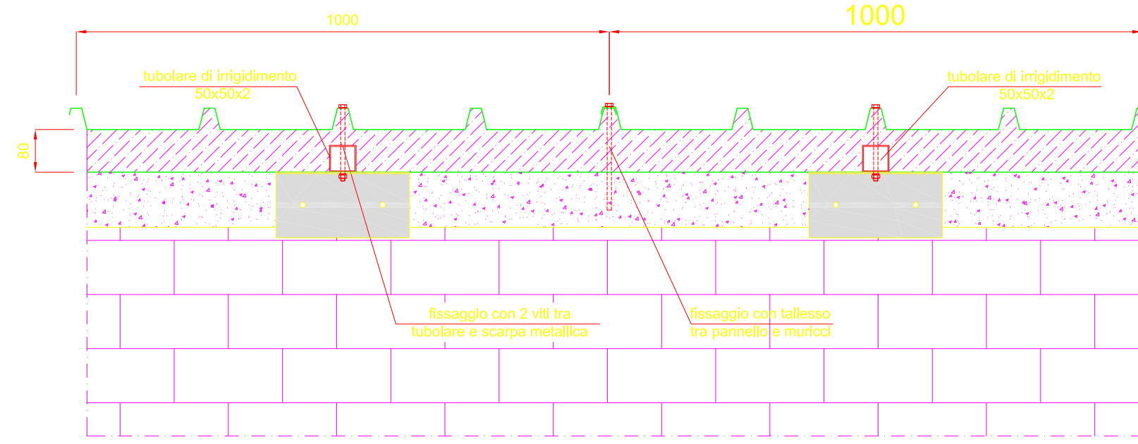
DETTAGLIO PANNELLI E VISTA SISTEMA DI FISSAGGIO (1:10)
