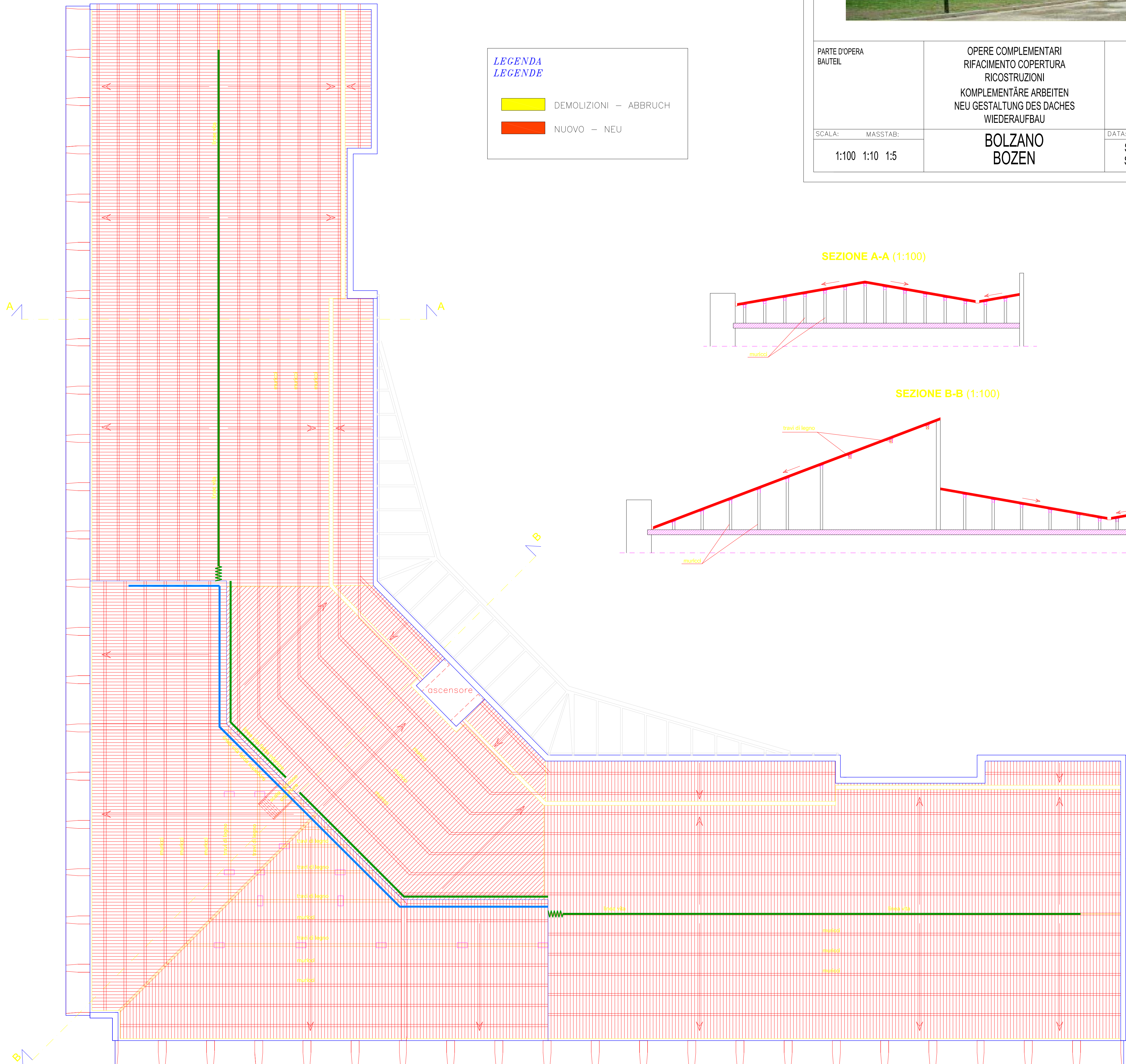
PIANTA (1:100)
