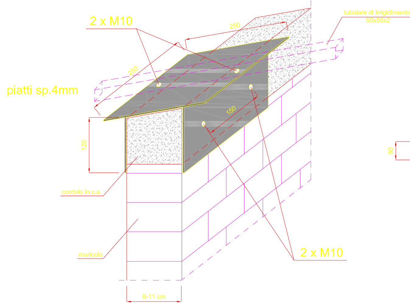
DETTAGLIO SCARPA METALLICA FISSAGGIO PANNELLI (1:5)
